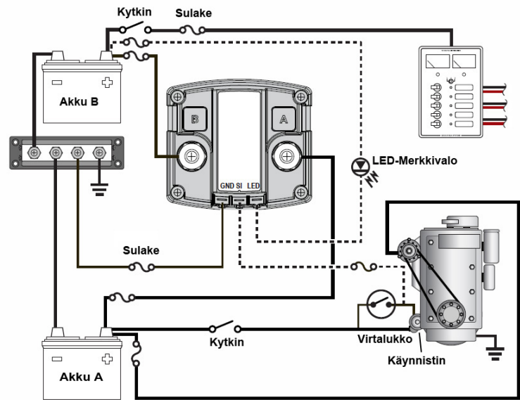
Tyypillinen 1100-0445 kaksoisakkureleen kytkentä
